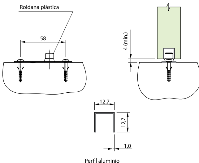
Perfil alumínio
