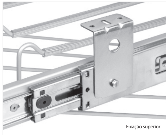
Montagem com suporte
