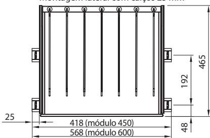
Dimensões definidas considerando MDF 15 mm
