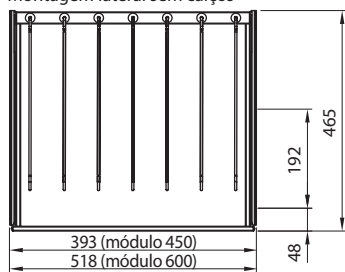
Montagem lateral com calços 25 mm
