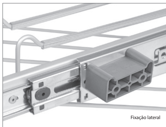
Montagem com calço
