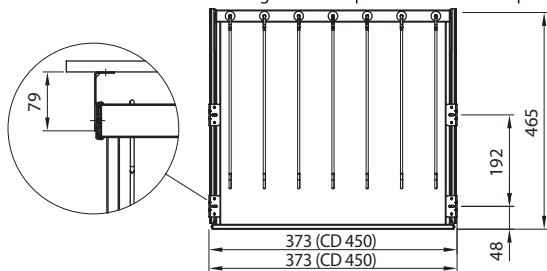
Montagem com suporte fixado sob tampo
