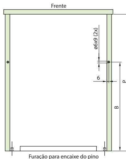
Furação para encaixe do pino
