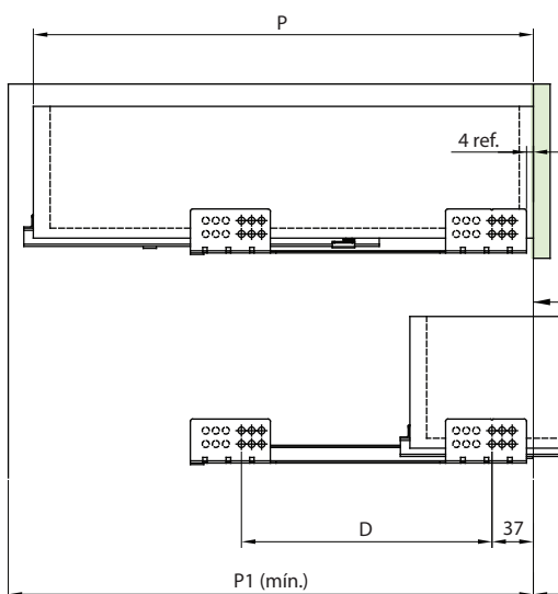
Dimensão para largura da gaveta
