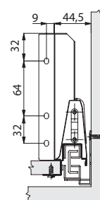
Posição Suporte para Traseiro de Madeira
