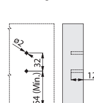
Furação conector no frontal da gaveta
